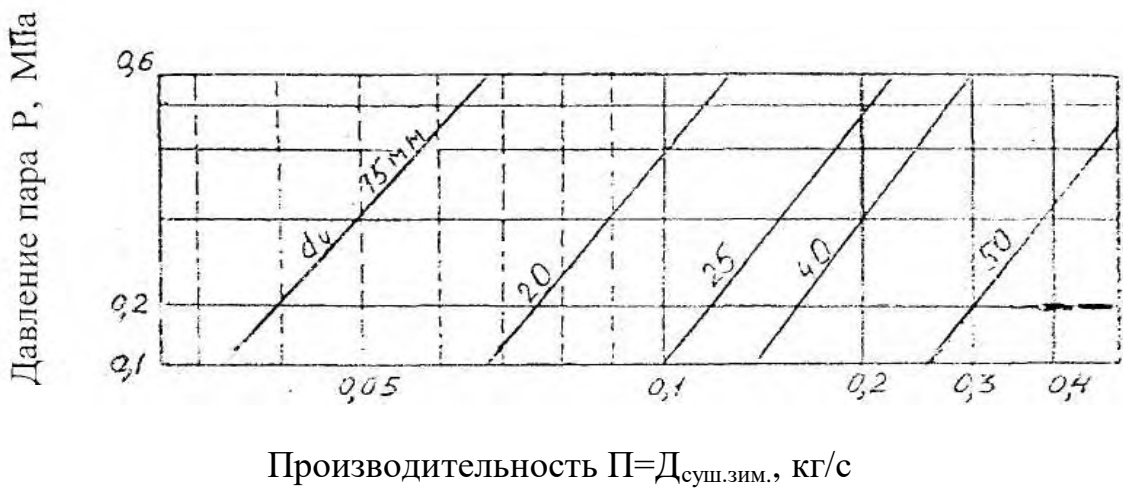
Рисунок Б.4 – Диаграмма для выбора диаметра условного прохода термодинамического конденсатоотводчика
